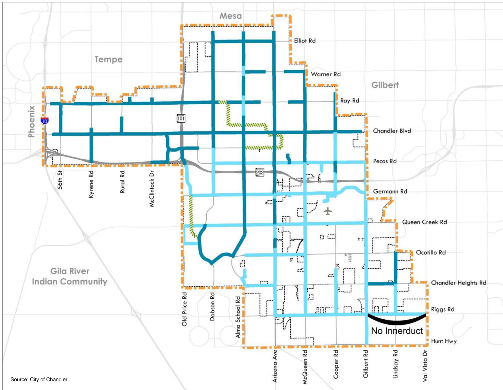
Figure 4-11. Existing Conduit Network
